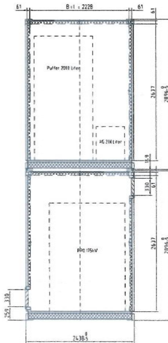
Schnitt G - G
