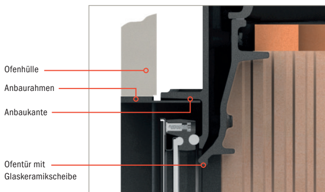
HKD 7: Tür bündig in Ofenhülle mit Anbaukante
